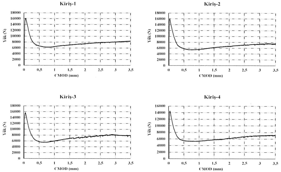
Şekil 1. Yük-Çatlak ağız deplasmanı açıklığı grafiği
