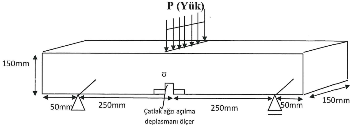
Şekil 1. Lif donatılı beton prizmalarda kullanılan numune geometrisi ve deney düzeneği
